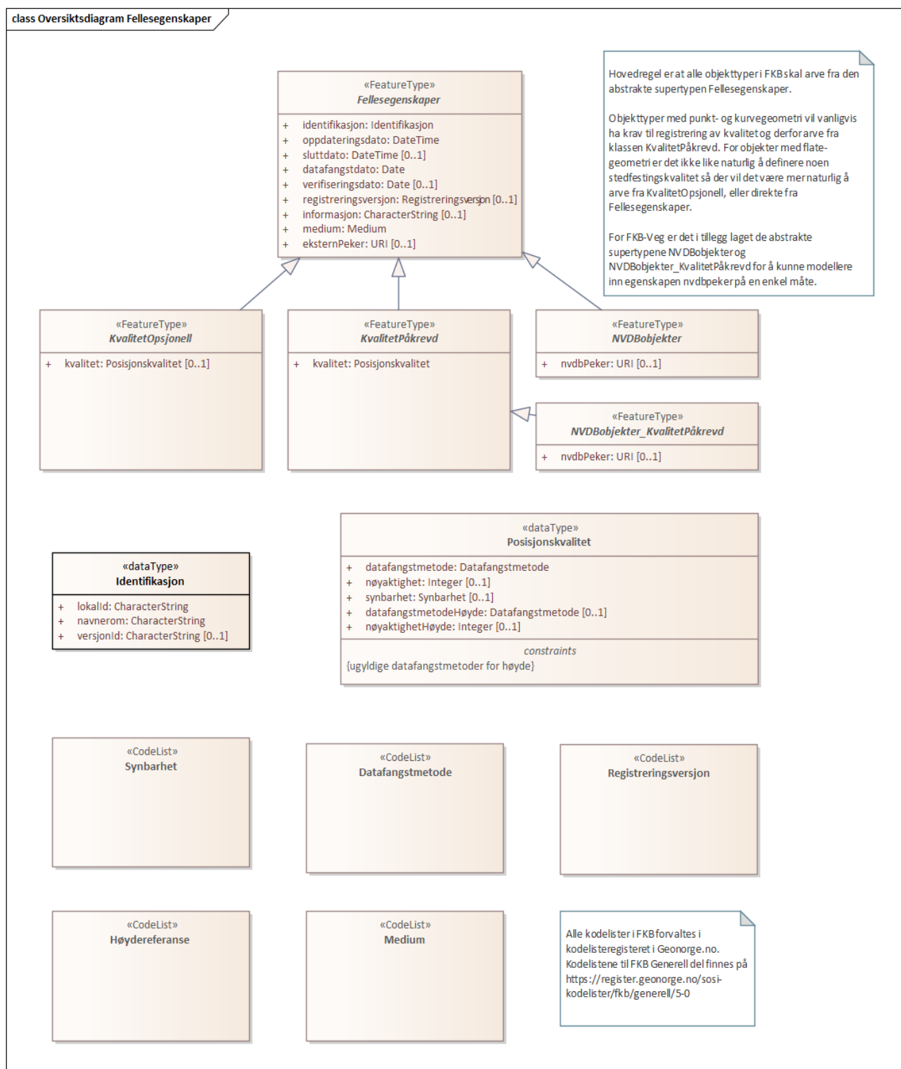
Figur 5. Oversiktsdiagram Fellesegenskaper
