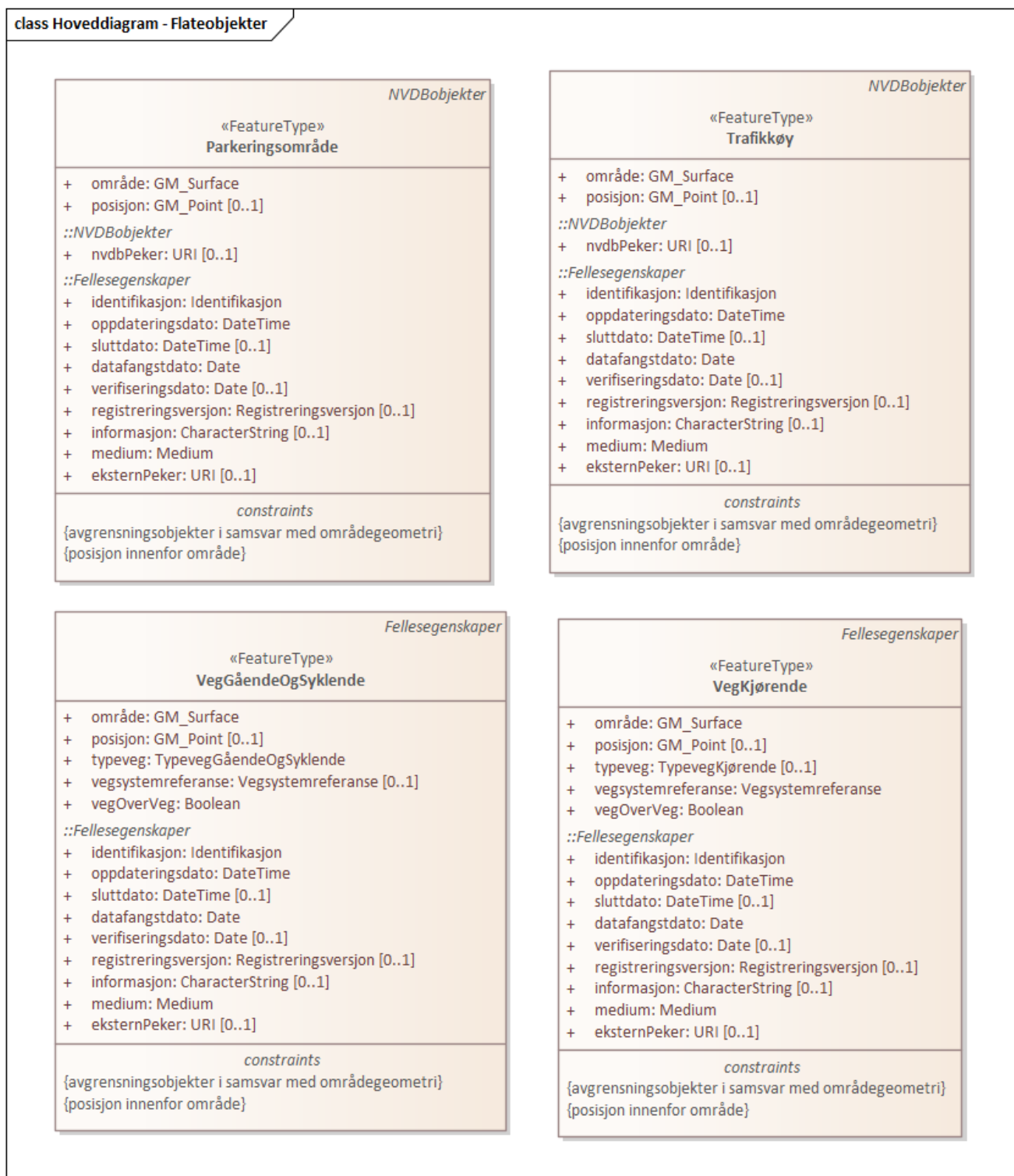
Figur 9. Hoveddiagram - Flateobjekter
