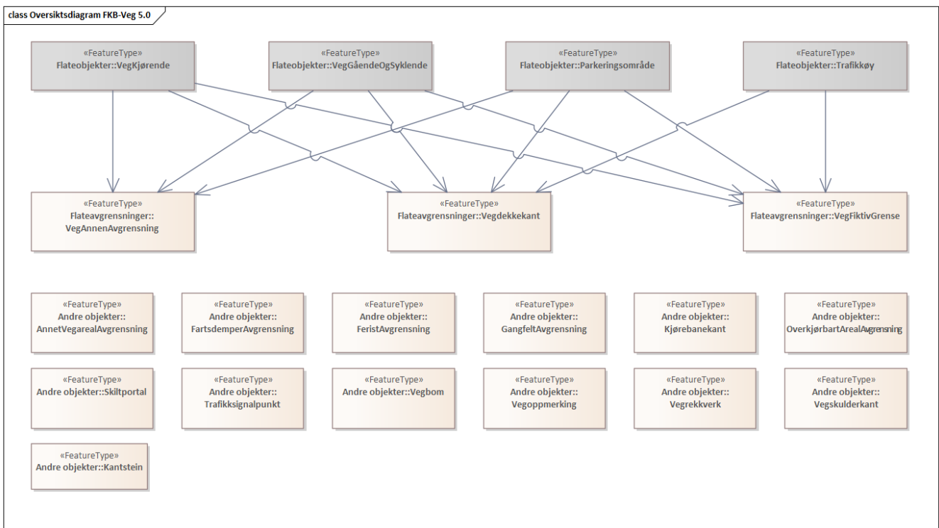
Figur 3. Oversiktsdiagram FKB-Veg 5.0
