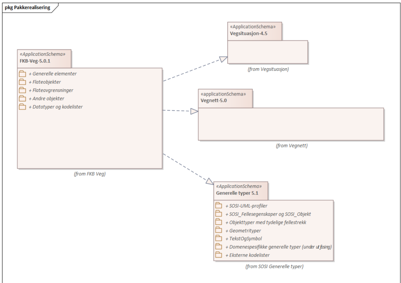
Figur 2. Pakkerealisering
